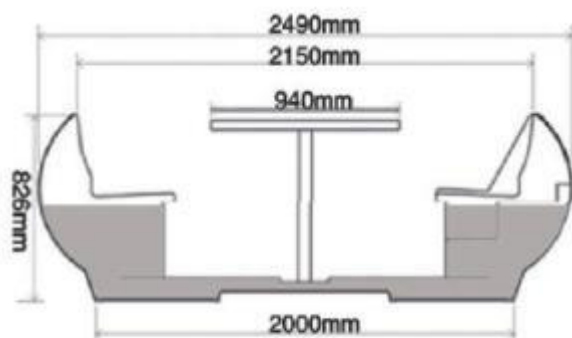
游艇内部聚氨酯发泡填充 Pufoam padding inside the boat
